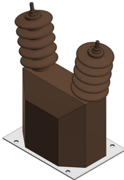
Figura 8. Modelo 3D de Transformador de tensión. Basado en Modelo VZF-36 de RITZ (RITZ Instrument Transformers).
