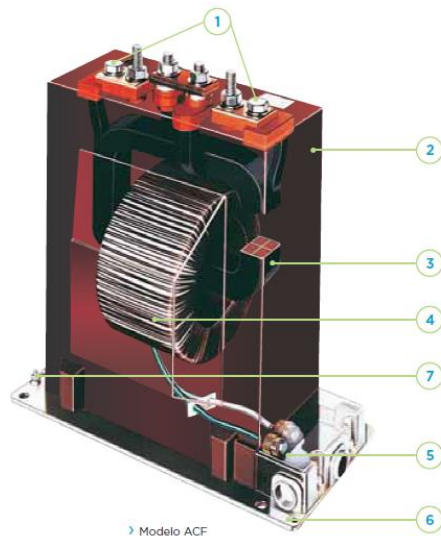
Figura 4. Transformador de corriente para media tensión de uso interior. Modelo ACF de ARTECHE (ARTECHE, ARTECHE - Catálogo Transformadores de Medida. Media Tensión Interior. Versión A1)
