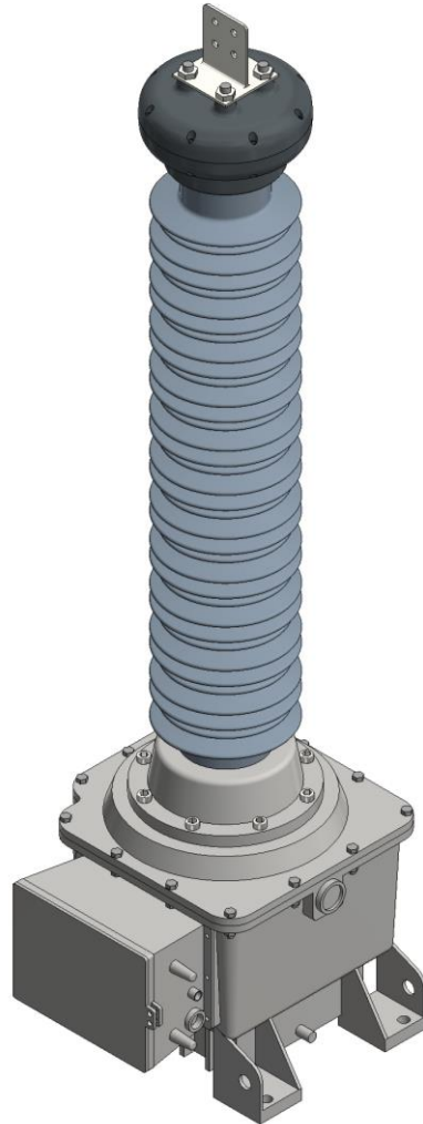
Figura 6. Modelo 3D de Transformador de tensión capacitivo, basado en modelo CPA de ABB (ABB Power technologies, 2005).
