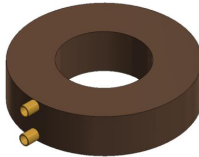
Figura 5. Modelo 3D de Transformador de corriente tipo venta para baja tensión de uso exterior. Basado en el Fabricante Rymel (RYMEL)
