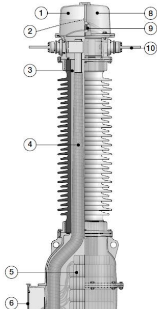
Figura 3. Transformador de corriente de uso exterior para media tensión Modelo IMB de ABB (ABB Power technologies, 2005)
