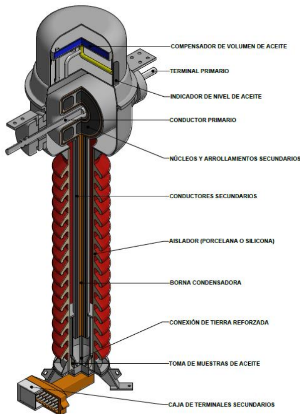
Figura 1. Modelo 3D de Transformador de corriente para alta tensión. Basado en el modelo CA del fabricante ARTECHE. (ARTECHE, ARTECHE - Catálogo Transformadores de Medida Alta Tensión. Versión B2)
