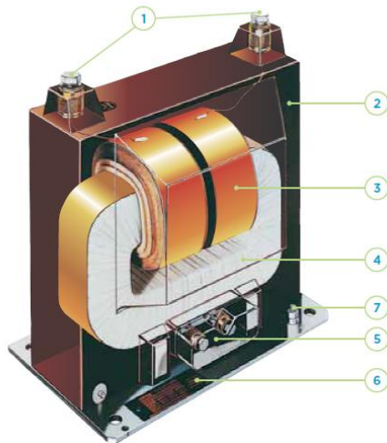
Figura 9. Transformador de tensión. Modelo VCL de ARTECHE (ARTECHE, ARTECHE - Catálogo Transformadores de Medida. Media Tensión Interior. Versión A1).
